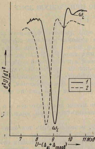
Рис. 1. Копии записей второй гармоники для образца Al — \text{Al}_2\text{O}_3 - \text{Pb}_{0,93}\text{In}_{0,07} при P = 9 (1) и P = 0 кбар (2)
